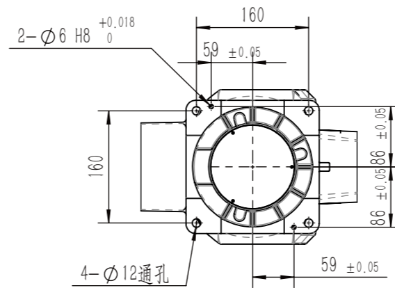
安装底座
